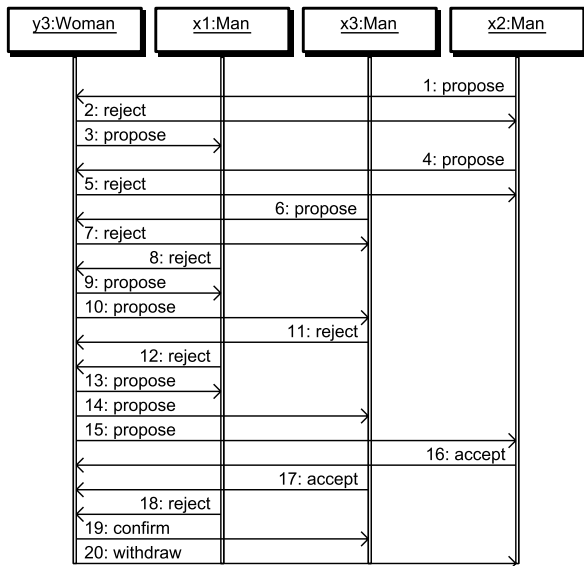
FIGURE 2 – Trace d'exécution de Casanova du point de vue de l'agent y_3
