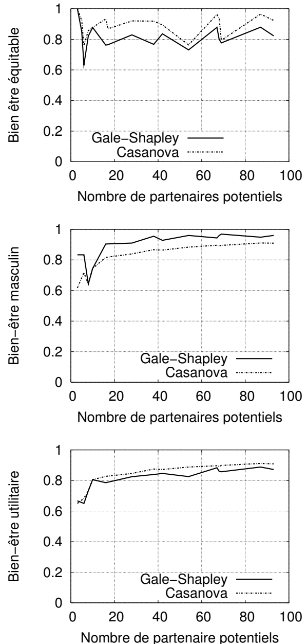
FIGURE 3 – Comparaison des solutions de Casanova avec celles de GS (ou DisEGS).
