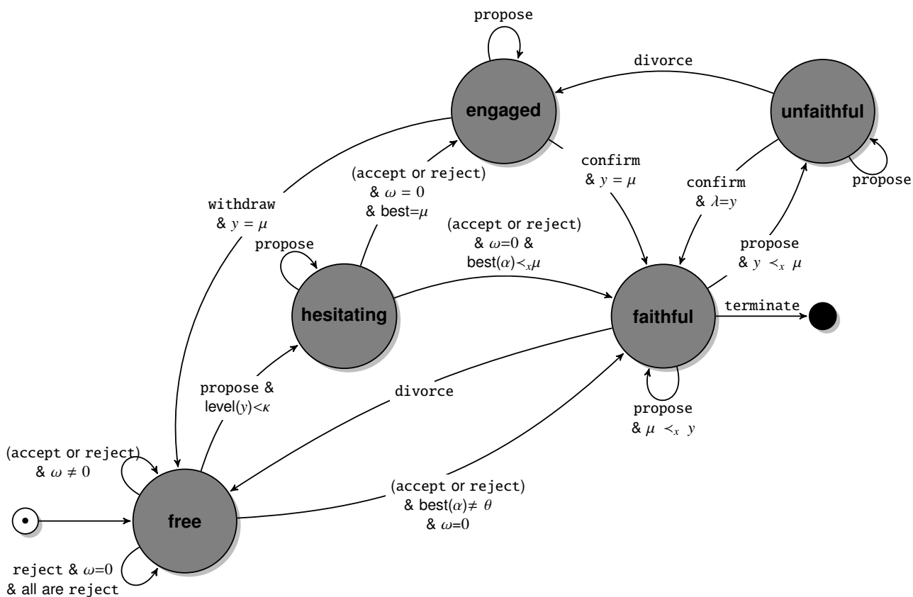
FIGURE 1 – Comportement des agents représenté comme un automate fini déterministe
